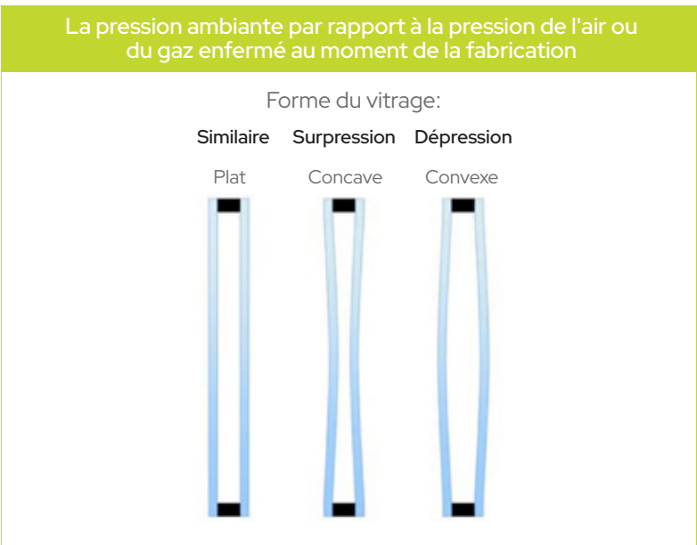
Figure 20 : Déformations des vitrages isolants dues aux variations de pression.
