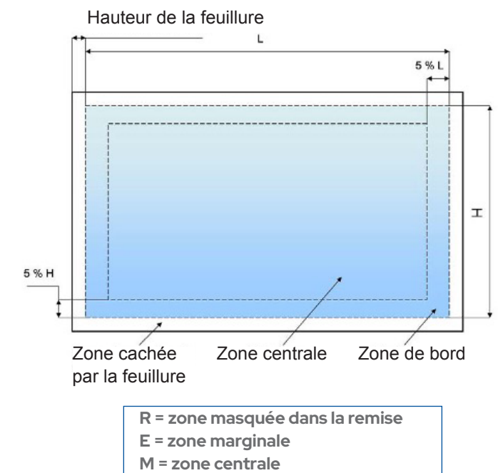
Figure 9: Les zones des vitrages
