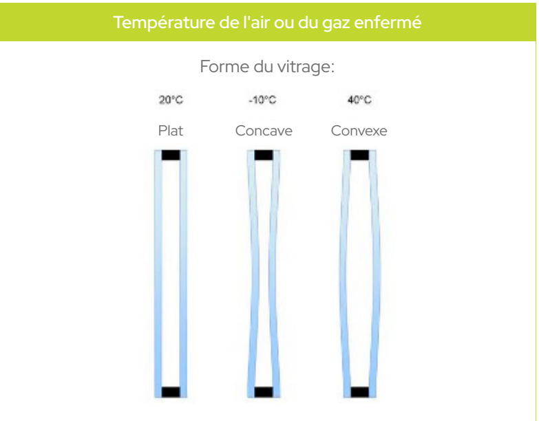
Figure 19 : Déformations des vitrages isolants dues aux variations de température.
