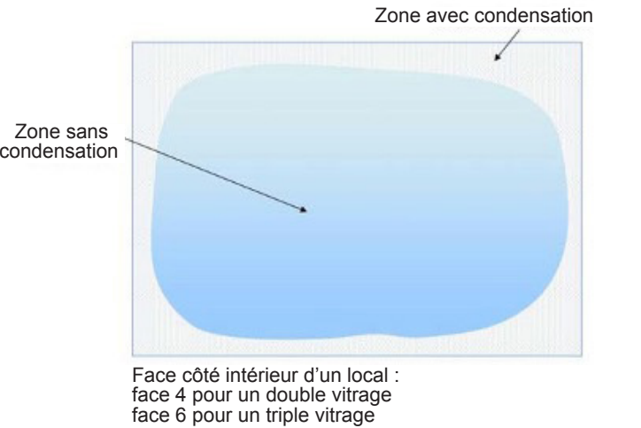
Figure 15 : Condensation sur face d'un vitrage côté intérieur d'un local.
