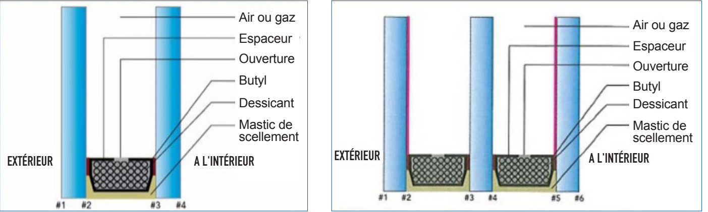
Figure 14 : Vitrage isolant : composition et numérotation des faces.
