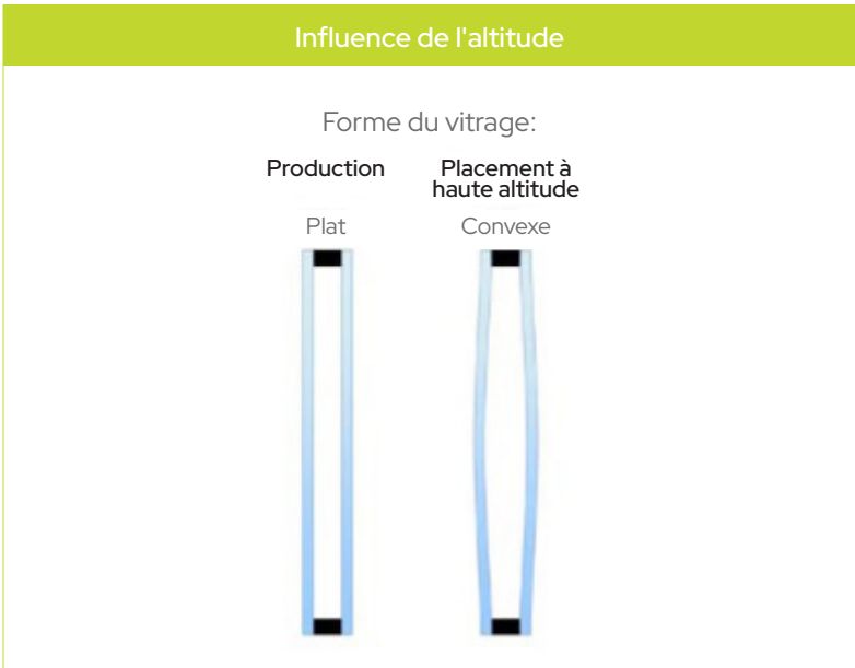
Figure 21 : Déformations des vitrages isolants dues aux variations d'altitude.
